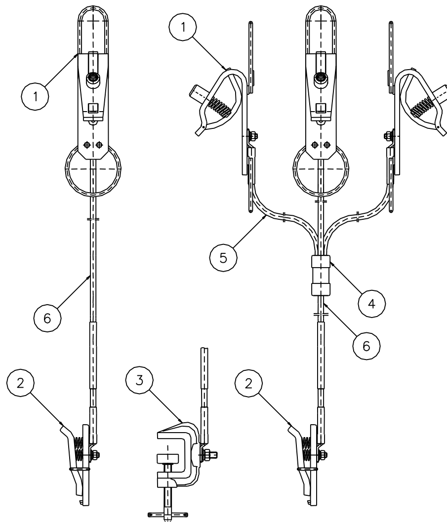
Uziemiacz U1-SD
